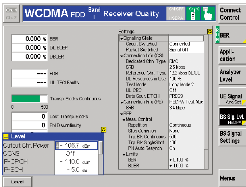
上图所示为在测试还回模式2下进行的P-CPICH为-110 dBm的UE接收机灵敏度测量。除最小DL功率条件之外，还可测试UE在压缩模式是否能够保持相同的灵敏度。R&S®CMU 200还提供“丢失传输数据块”计数，大大方便了错误检测。
